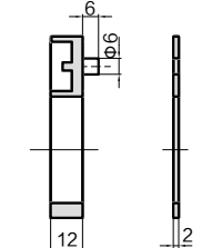
SK19-PE12底座 Pedestal 垫片 Cushion
