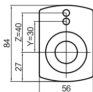
定位销位置Y或Z Torque pin position Y or Z
